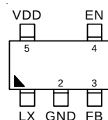
TSOT-23-5
