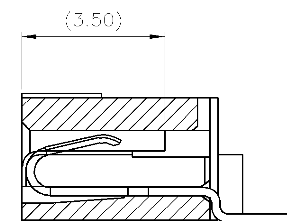
SECTION A-A
