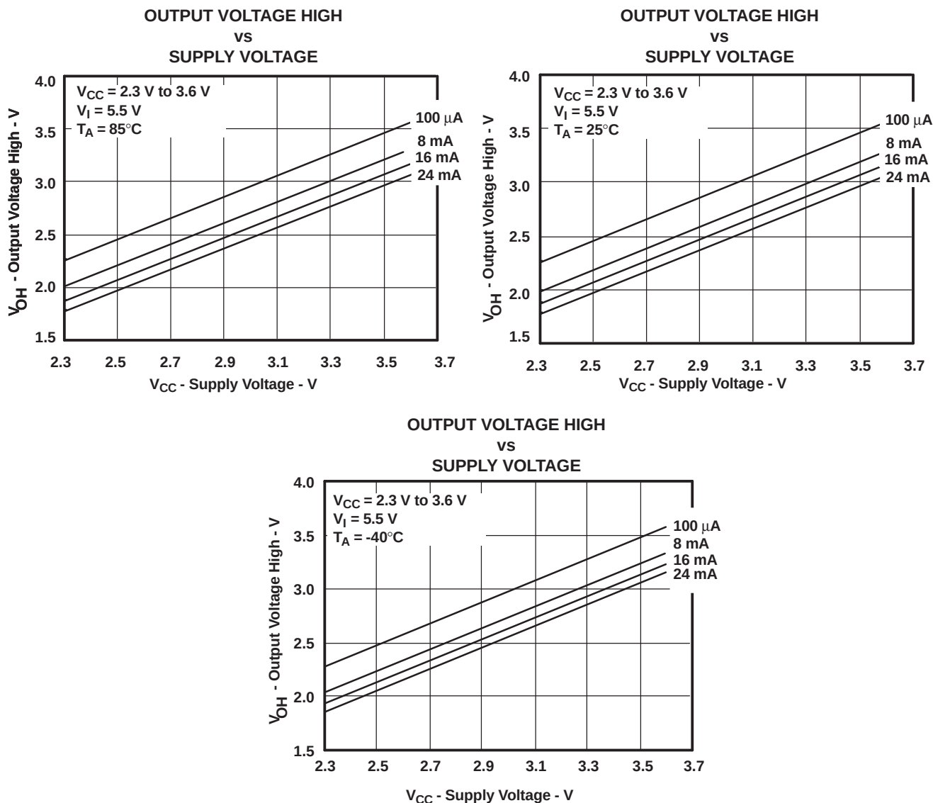
Figure 4. V_{OH} Values
