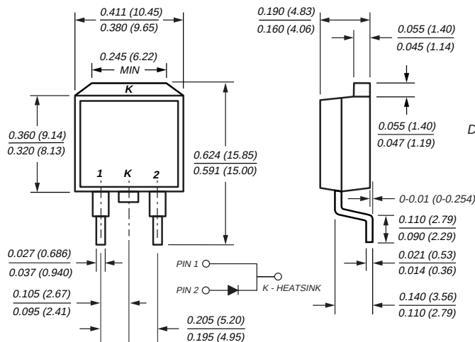
TO-263AB
