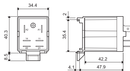
065.07 avec relais monté
