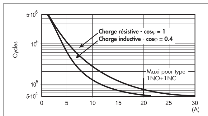
F 65 - Durée de vie électrique (AC) en fonction de la charge
