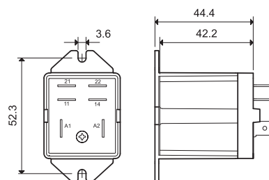
065.05 avec relais monté
