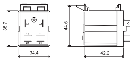
065.08 avec relais monté
