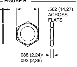
Hex Nut
