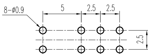
安装孔 PIERCING PLAN
