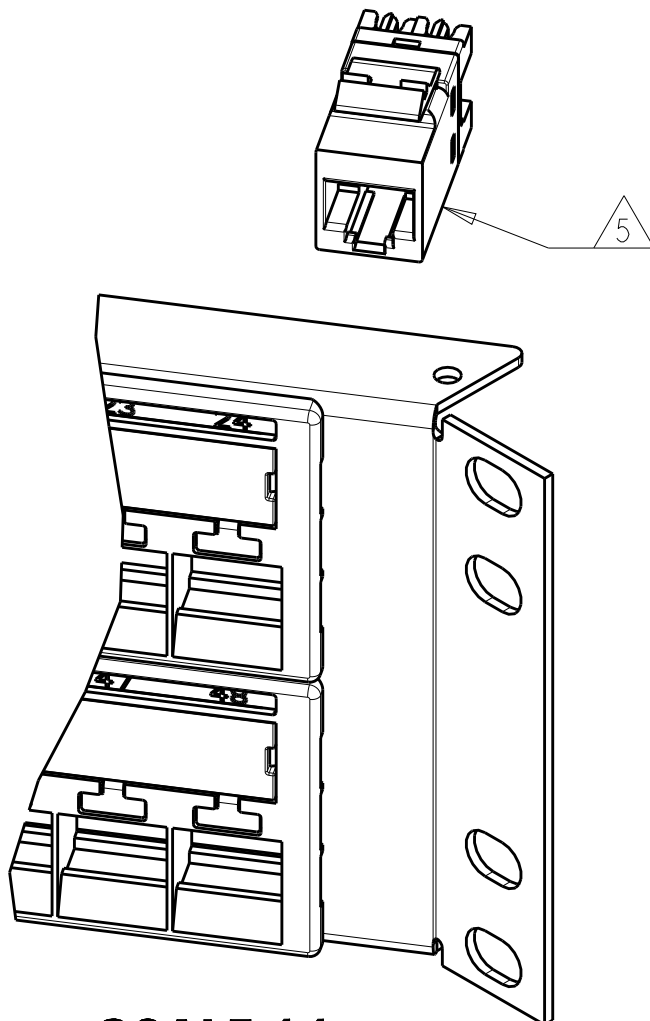
SCALE 1:1
