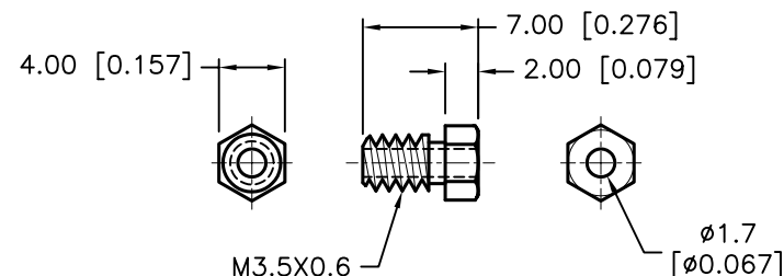
INTERNAL STUD
