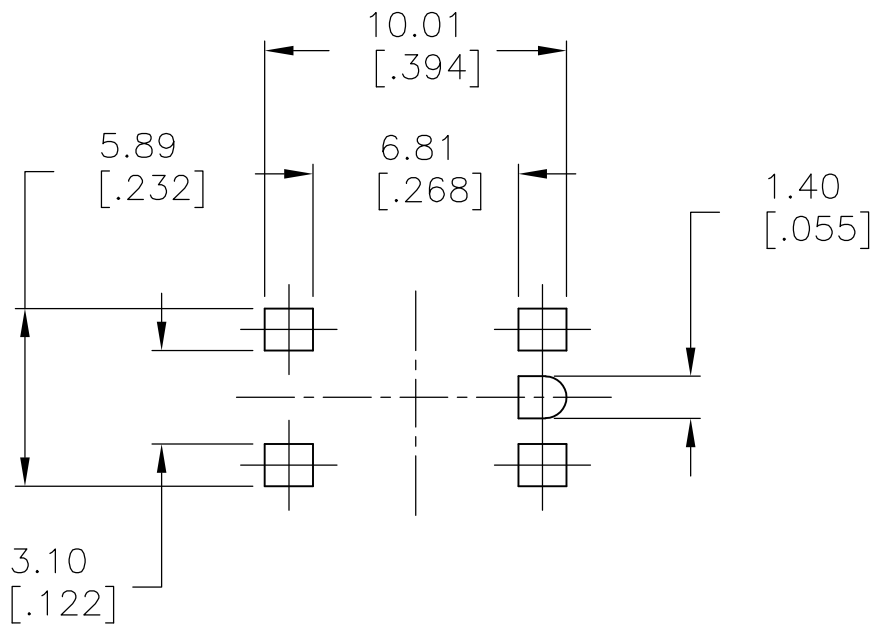
P.C.B. FOOTPRINT
