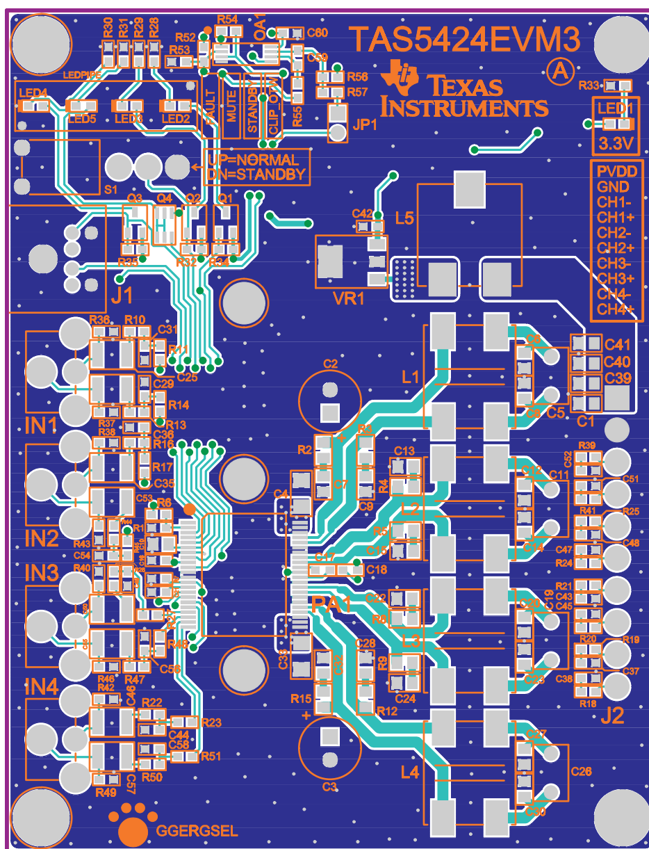
Figure 1-12. TAS5424AEVM3 Top Composite Layer
