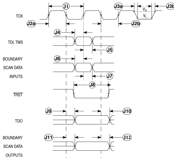
IEEE 1149.1 (JTAG) Timing
