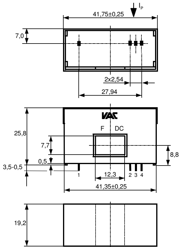
Maßbild Nr. 1
