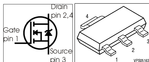
PG-SOT223
