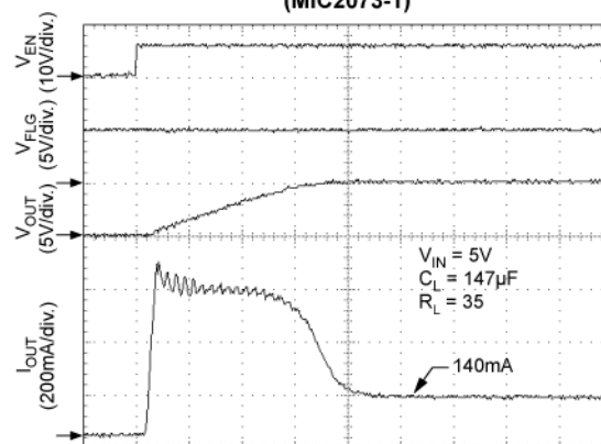
Turn-On (MIC2073-1)
