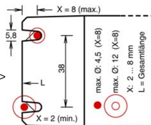
Befestigungs-Maße
