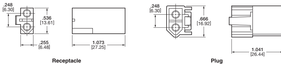
Receptacle
