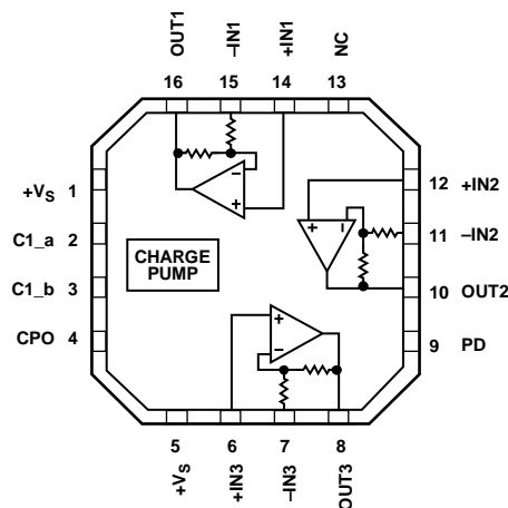
ADA4859-3
