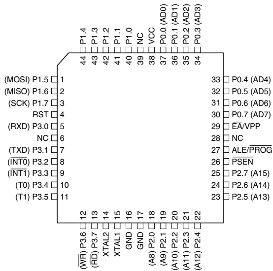
TQFP
