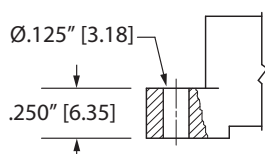
FLUSH MOUNTING (D)
