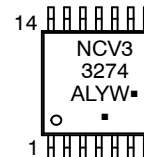
TSSOP-14 DTB SUFFIX CASE 948G
