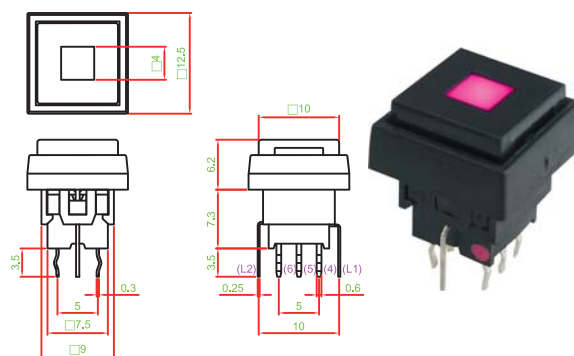
PS004-L22NPR1AXT□□□□
