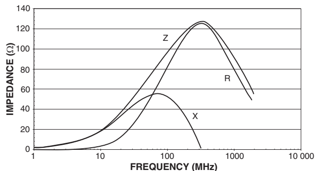
ILBB-0805 100 \Omega
