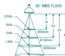
Superia 50 / 50W / 38°
