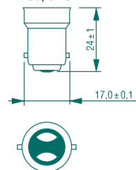
B15d/SBC
