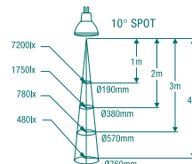
Superia 50 / 35W / 10°
