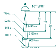
Superia 50 / 35W / 10°
