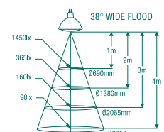
Superia 50 / 35W / 38°
