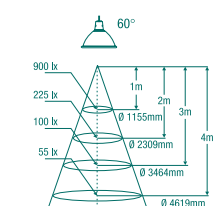
Dichroic 50W / 60°
