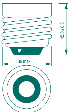
E40/GES
