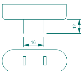
Gx16d
