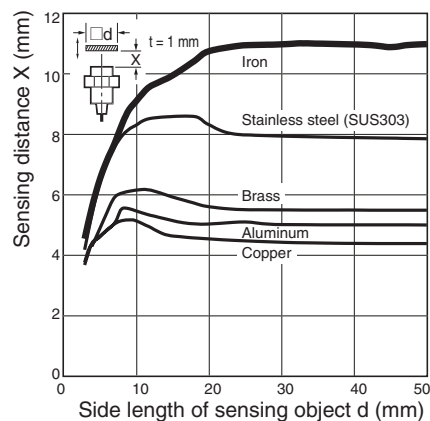
E2A3-M18KS11
