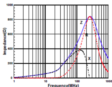
ACML-0402H-601
