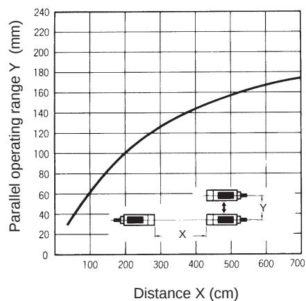
E3S-5E4(41)(42)
