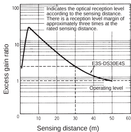
E3S-DS30E4S(1)
