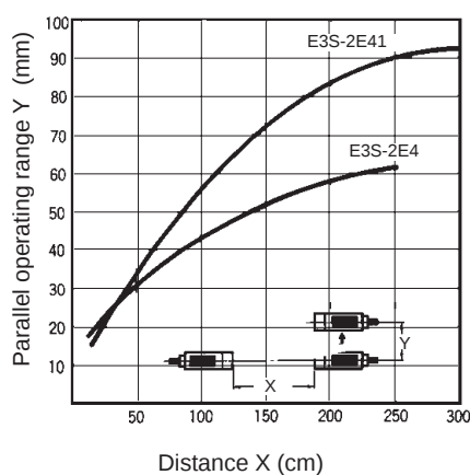
E3S-2E4(1)
