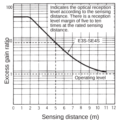
E3S-5E4S(1)
