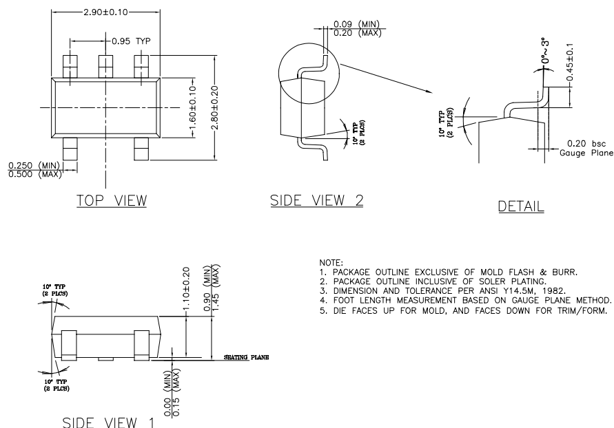
SOT-23-5 (M5)
