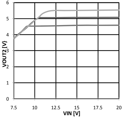
Fig.18 VIN-VOUT2
