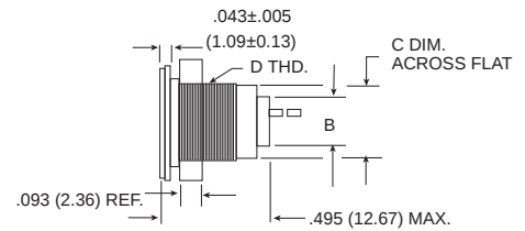
Receptacle
