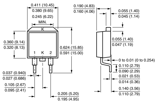
TO-263AB
