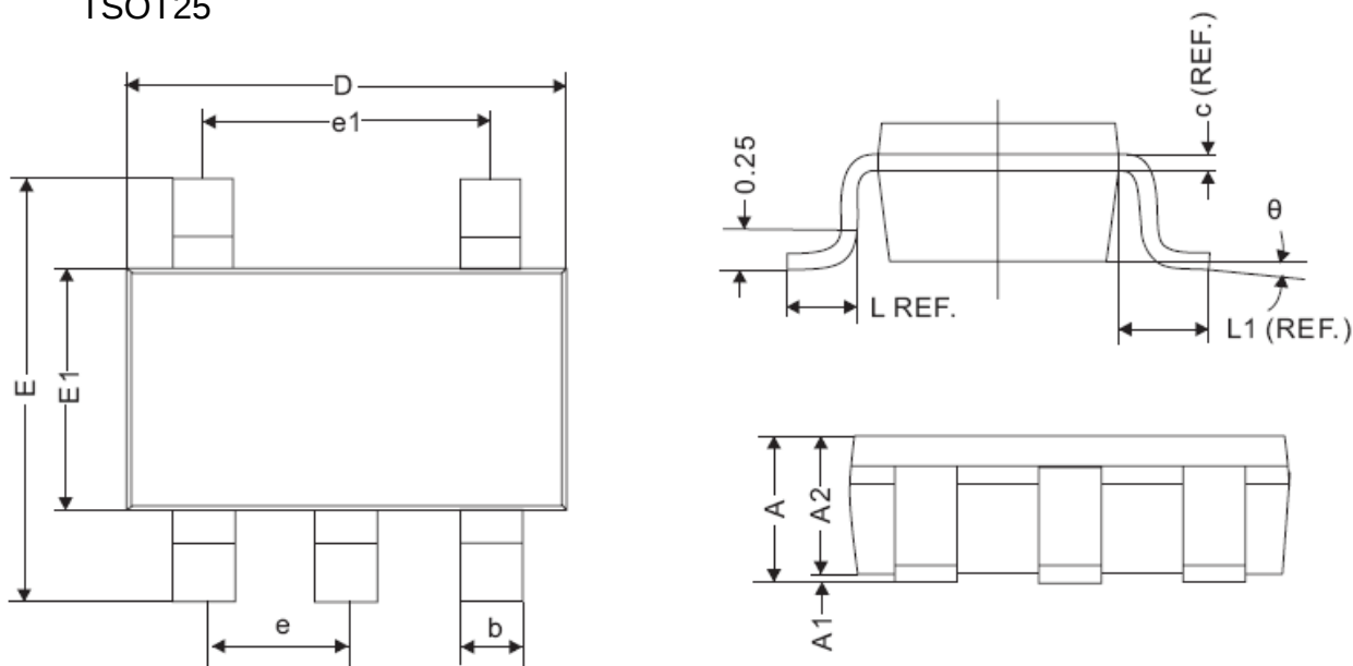
TSOT25
