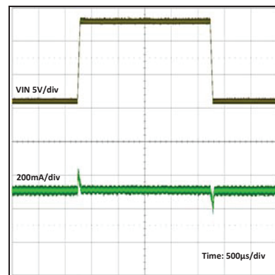
6-18 V Fast VIN Transient
