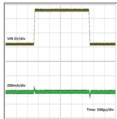
6-18 V Fast VIN Transient
