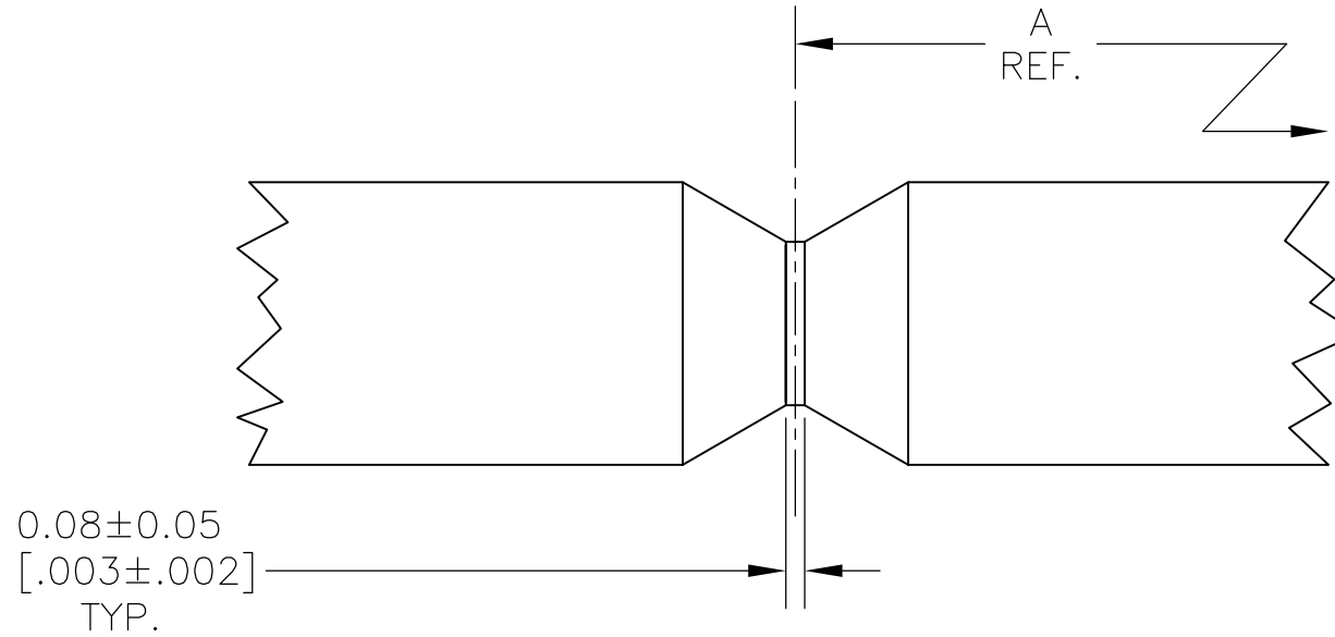
DETAIL W 30:1
