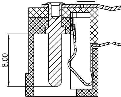
SEC: A-A
