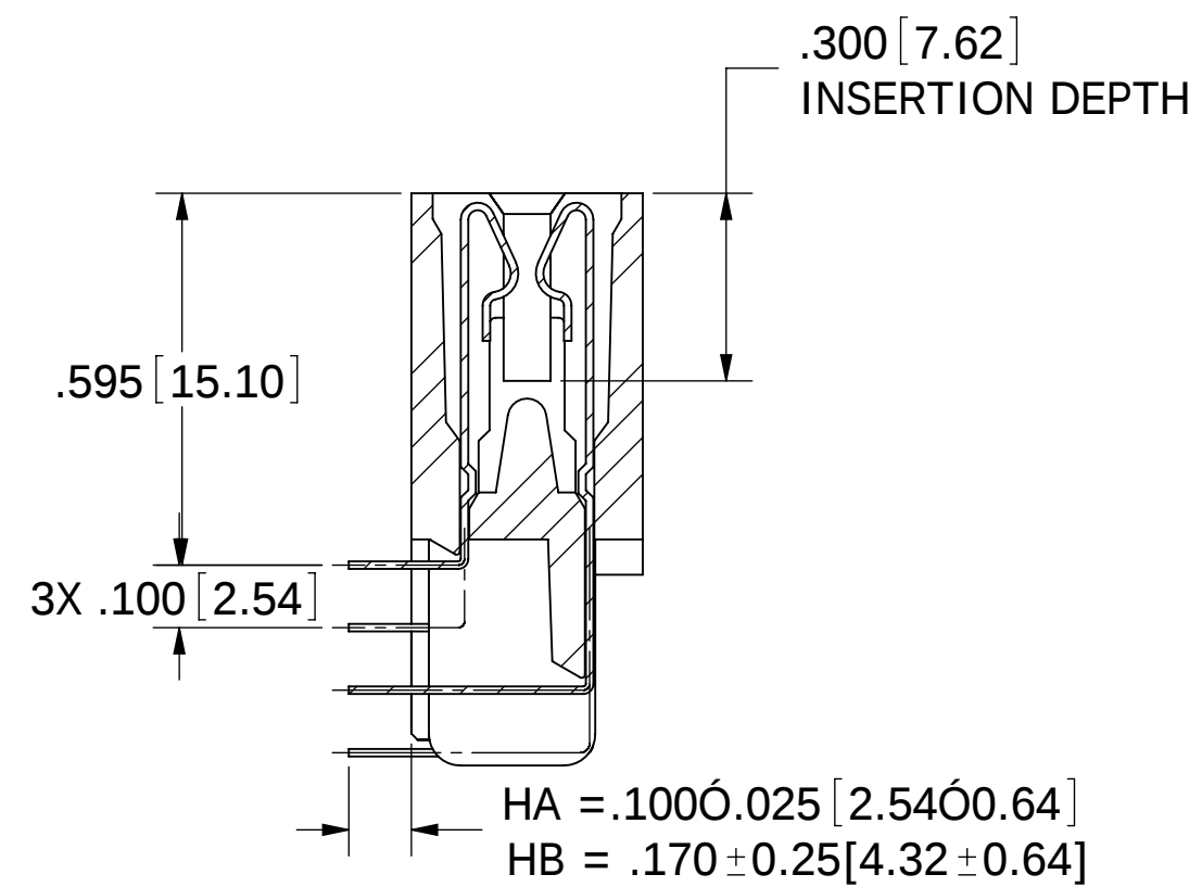
SECTION A-A SCALE 3 : 1
