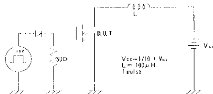
図1 測定回路
