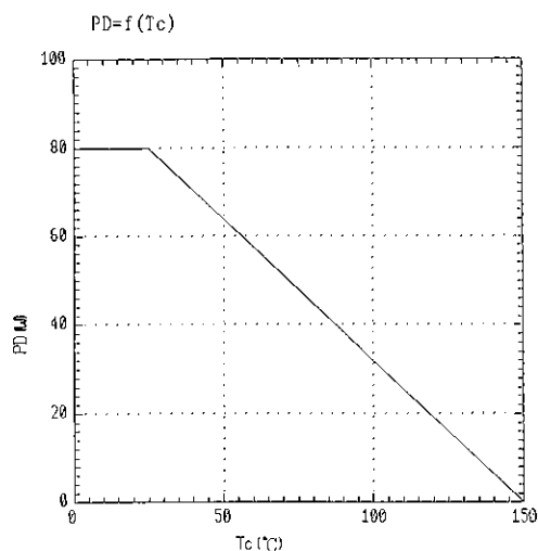
電力損失 Power Dissipation
