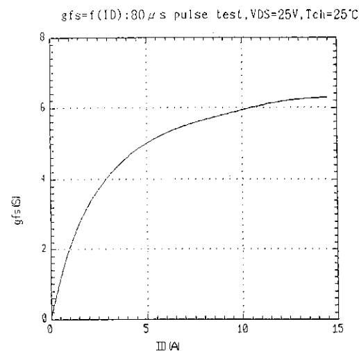
伝達コンダクタンス Typical transconductance
