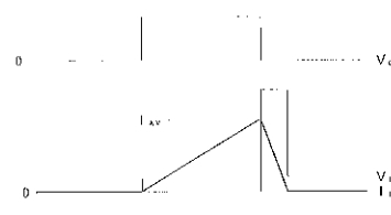
図2 動作波形
