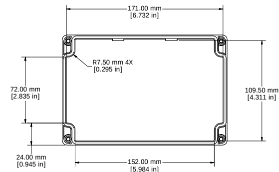
LID - INSIDE
