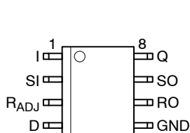
SO-8
