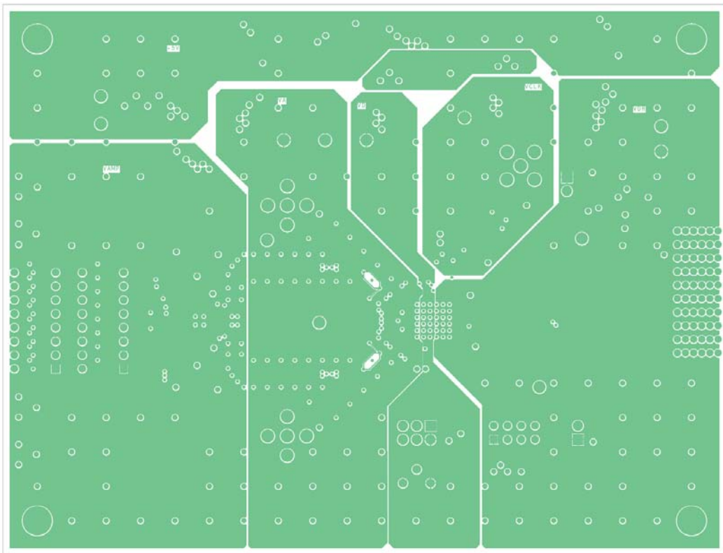
Layer 4 : Power
