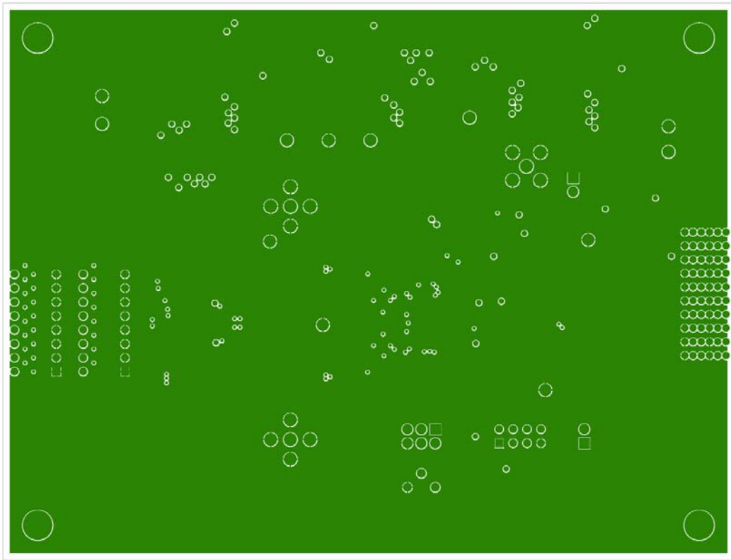
Layer 3 : Ground
