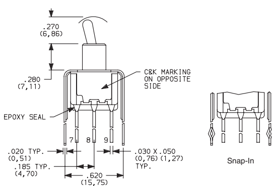
Actuator Shown In Pos. 1
