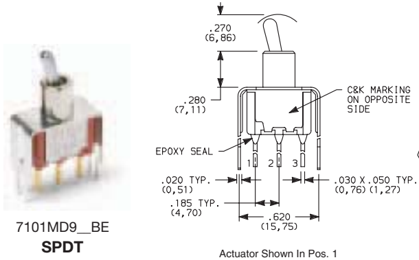
Actuator Shown In Pos. 1
