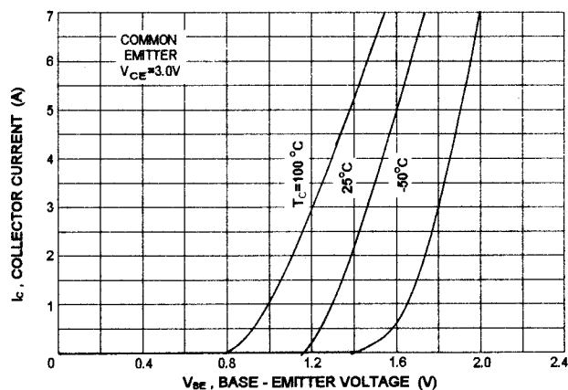
I_C - V_{BE}
