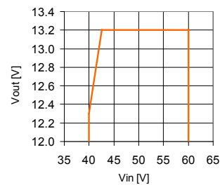
Vin range:40-60Vdc
