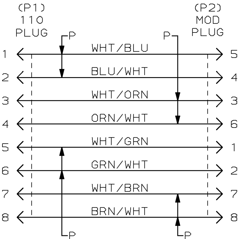
WIRING DIAGRAM T568A
