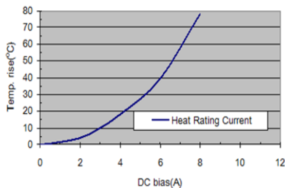
ASPI-0630HI-6R8
