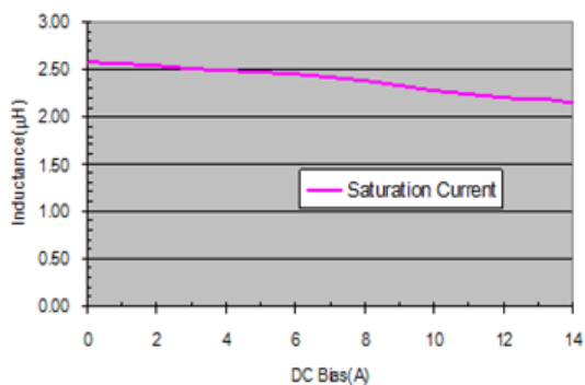
ASPI-0630HI-3R3
