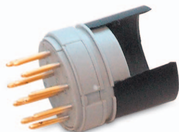
M23 Signalsteckverbinder Serie RF sind jetzt in den Polzahlen 6 bis 17 verfügbar. Die Abbildung zeigt den 12-poligen Kabel- und Kupplungssteckverbinder mit Lötanschluss.
