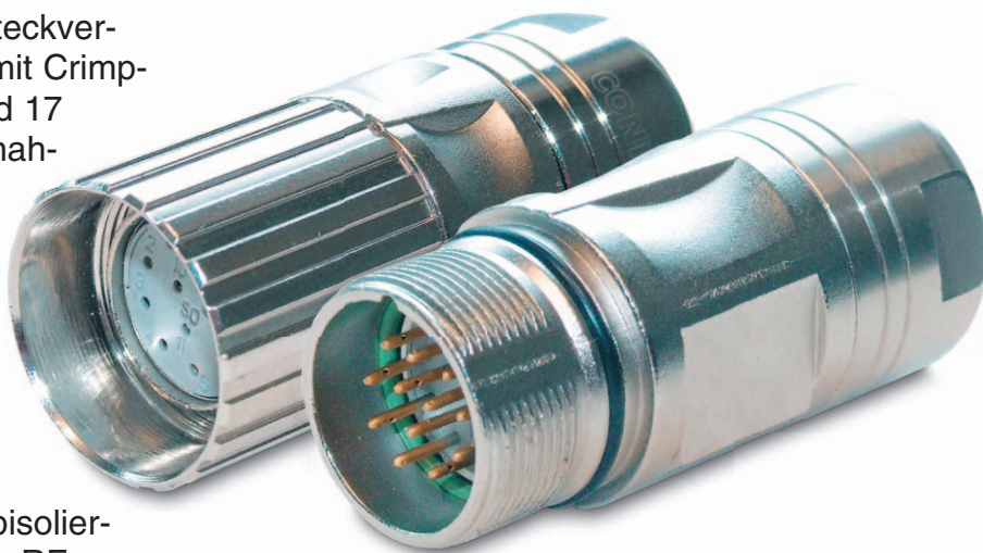
M23 Signalsteckverbinder Serie RF sind jetzt in den Polzahlen 6 bis 17 verfügbar. Die Abbildung zeigt den 12-poligen Kabel- und Kupplungssteckverbinder mit Lötanschluss.
