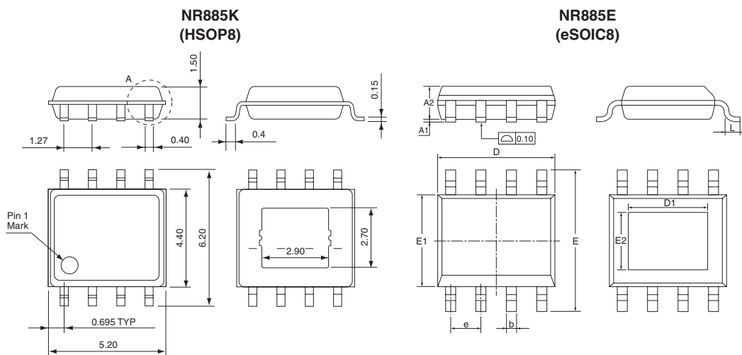
External Dimensions (NR885E)
