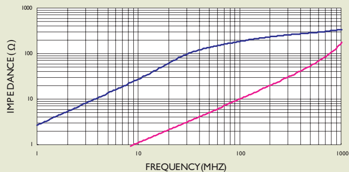
SBCB656030T-181-S
