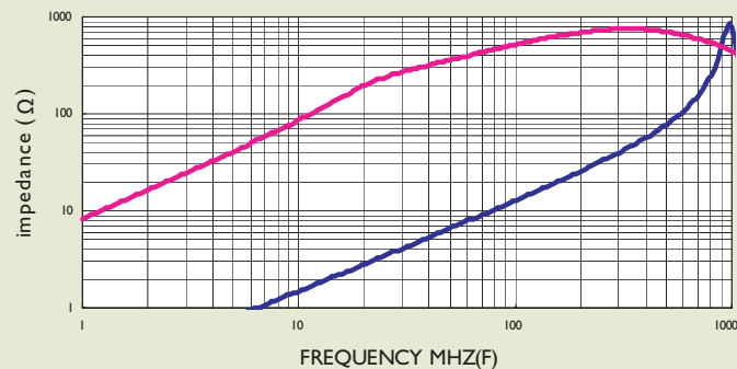
SBCB656030T-601-S
