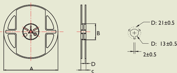
Reel Dimensions
