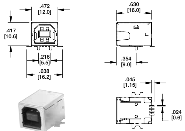
USB-B-S-R-TSMT
