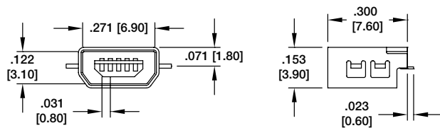
MUSB-AB-S-RA-TSMT
