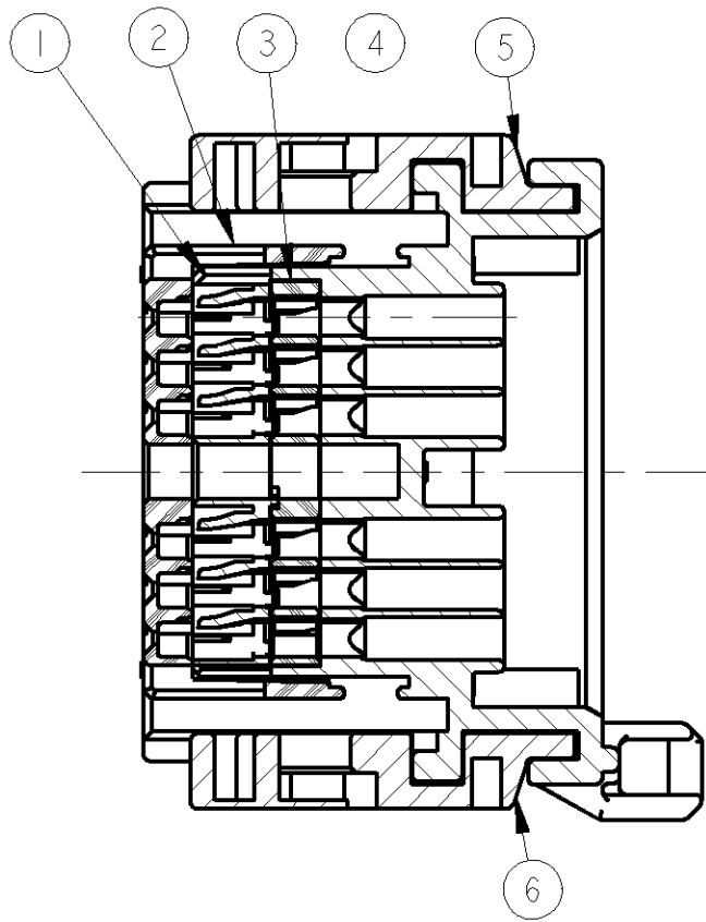
A - A
